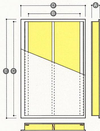
■商品寸法図
